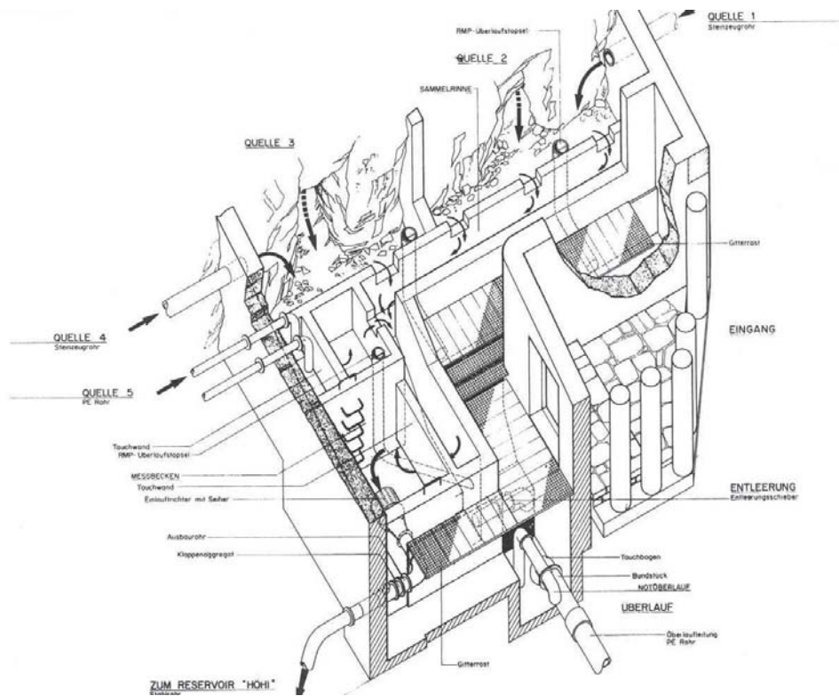
Isometrische Darstellung
